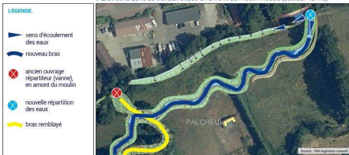
PLAN de la zone de travaux située en amont du moulin Robbe (secteur vanne)
